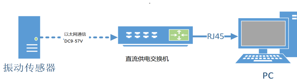
图 3 直流供电交换机连接示意图
