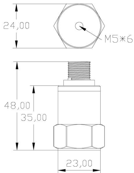
图 3 产品外形及安装尺寸图
